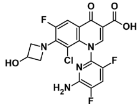
Şekil 1. Delafloksasin: 1-(6-Amino-3,5-difloropiridin-2-il)-8-kloro-6-floro-7-(3-hidroksiazetidin-1-il)-4-oksokinolin-3-karboksilik asit.
