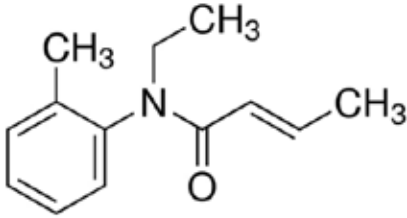
Şekil 3. Krotamiton: N-Etil-N-(2-metilfenil)-2-bütenamit.
